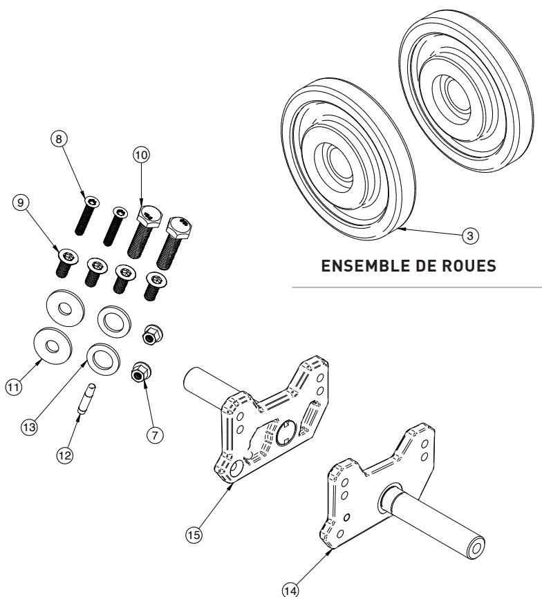
ENSEMBLE D'ADAPTATEUR STRYKE
