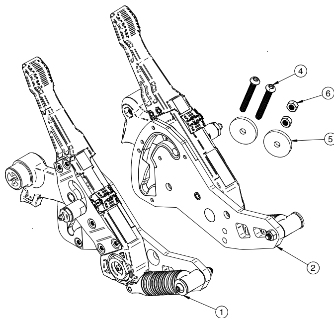
ENSEMBLE MÉCANISME ROUSKI EVO
