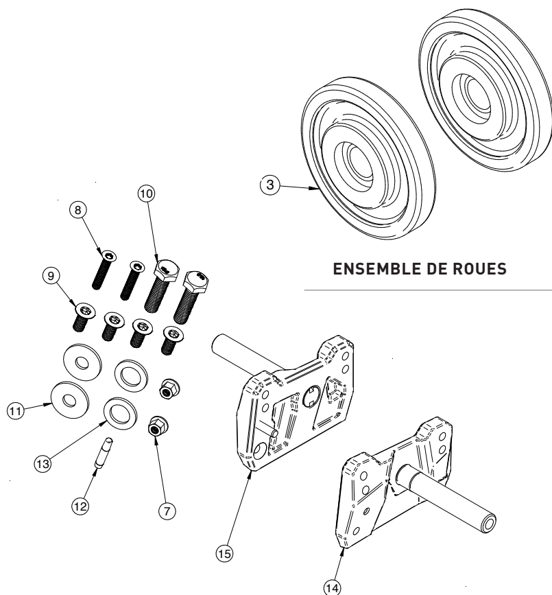
ENSEMBLE D'ADAPTATEUR PILOT 5.7
